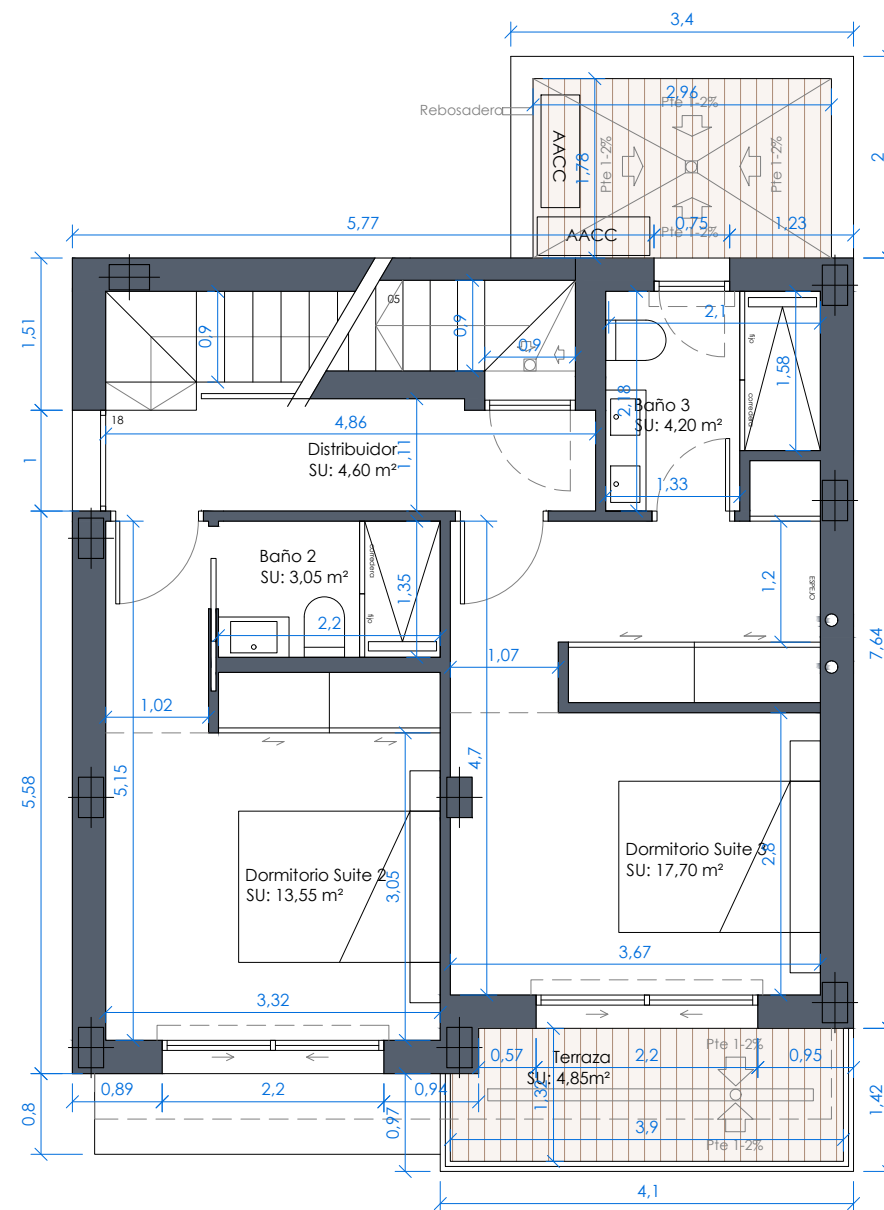
PLANTA PRIMERA
