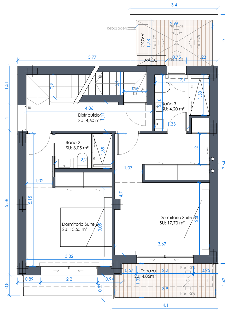
PLANTA PRIMERA
