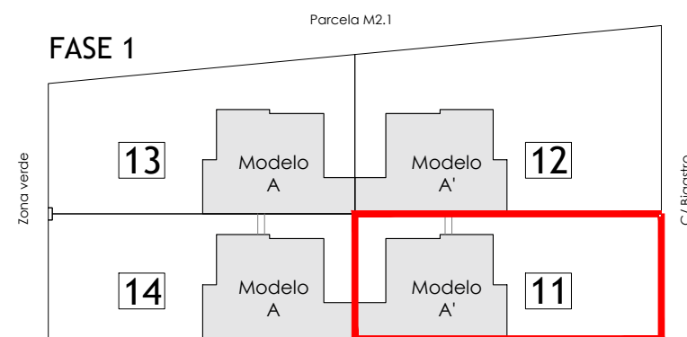
PLANTA CUBIERTA
