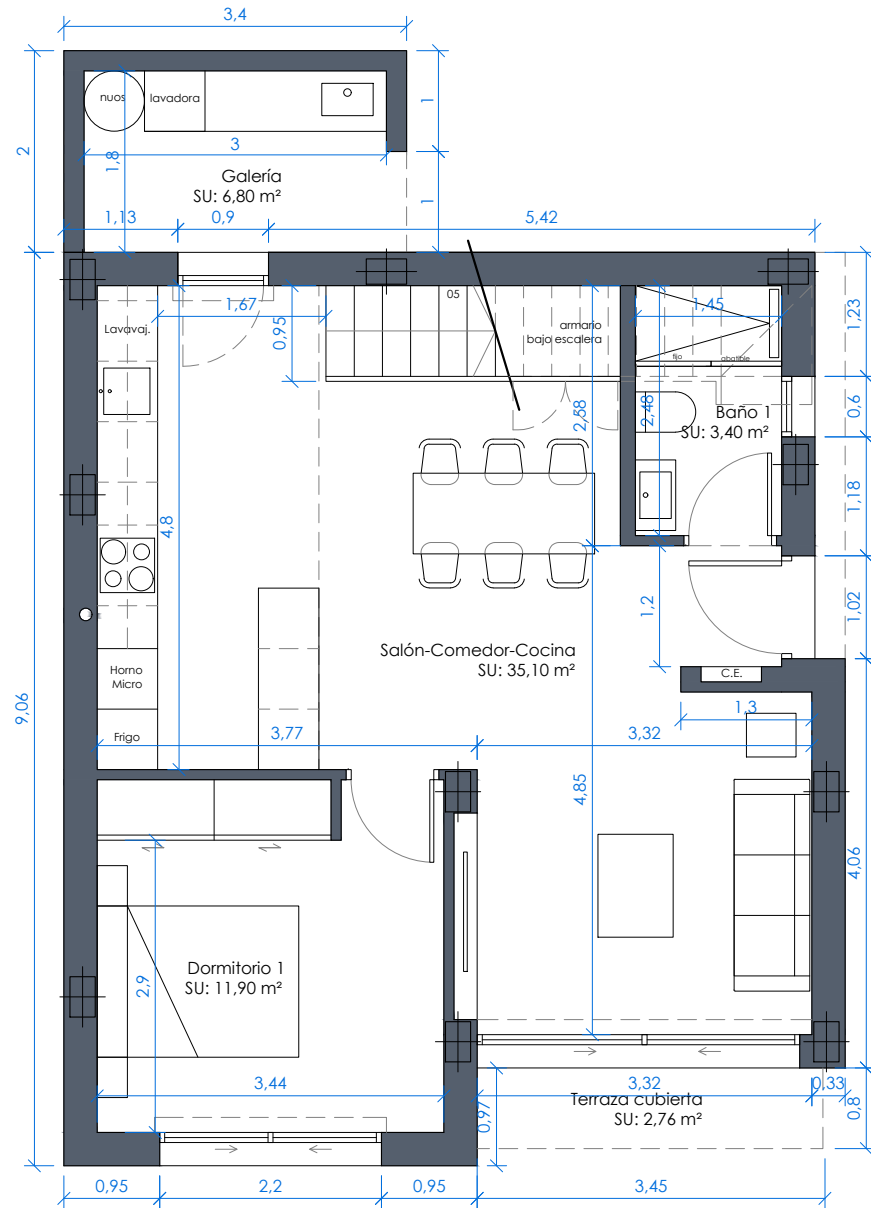
PLANTA BAJA
