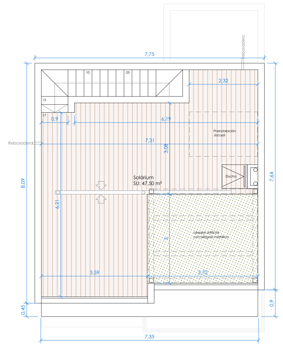
PLANTA CUBIERTA
