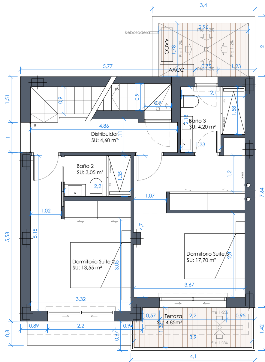
PLANTA PRIMERA
