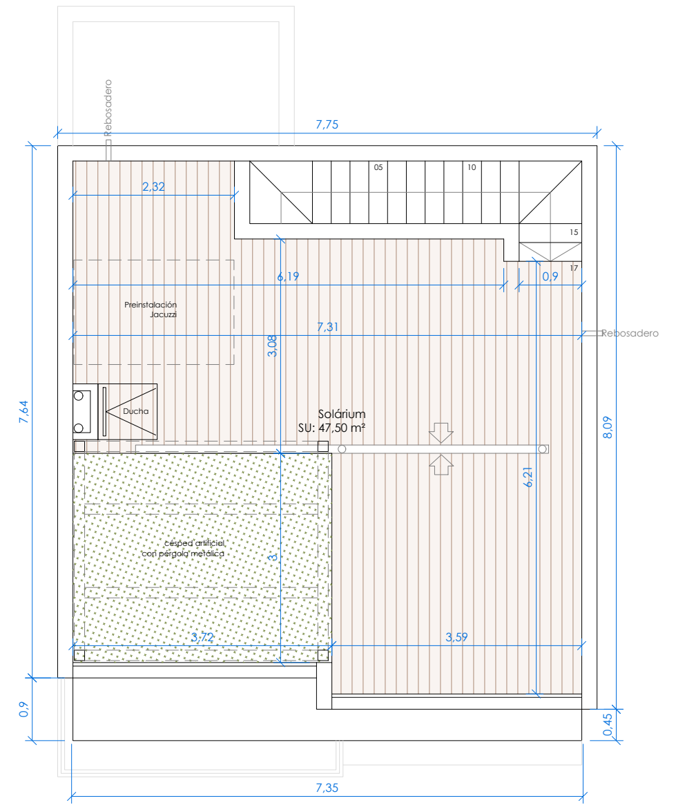
PLANTA CUBIERTA
