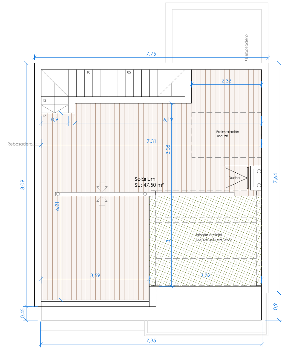
PLANTA CUBIERTA
