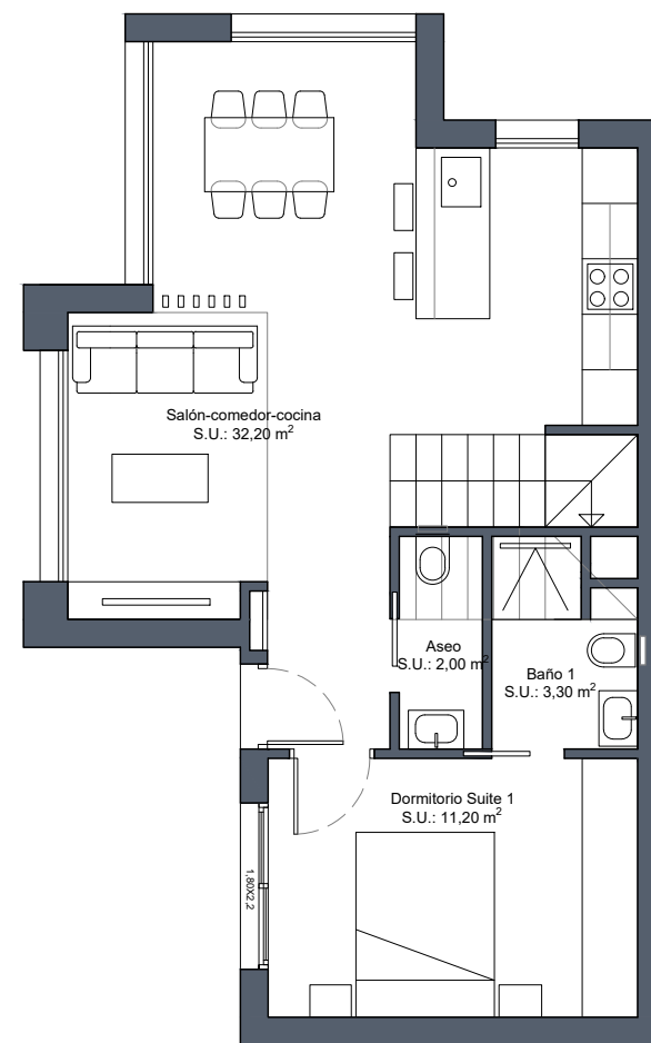
Planta baja
