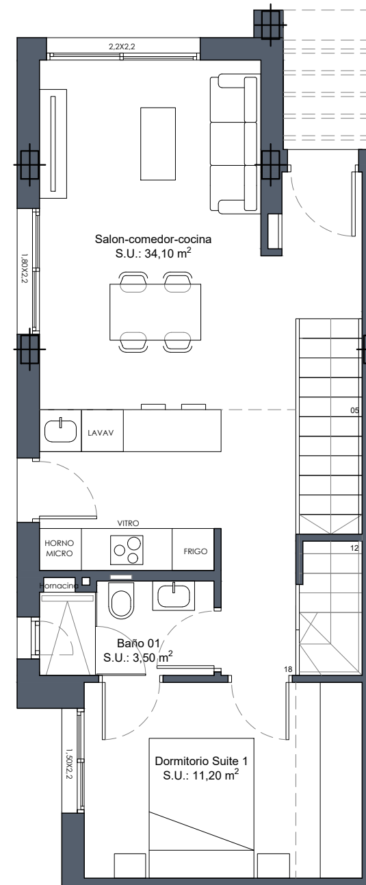
Planta baja
